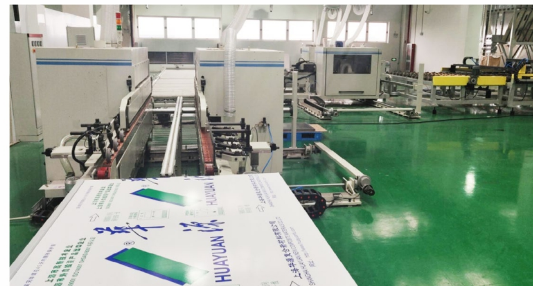
大型数控专业开槽机 CNC Slotting Machine
